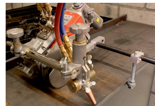
Plate edge guide roller option
